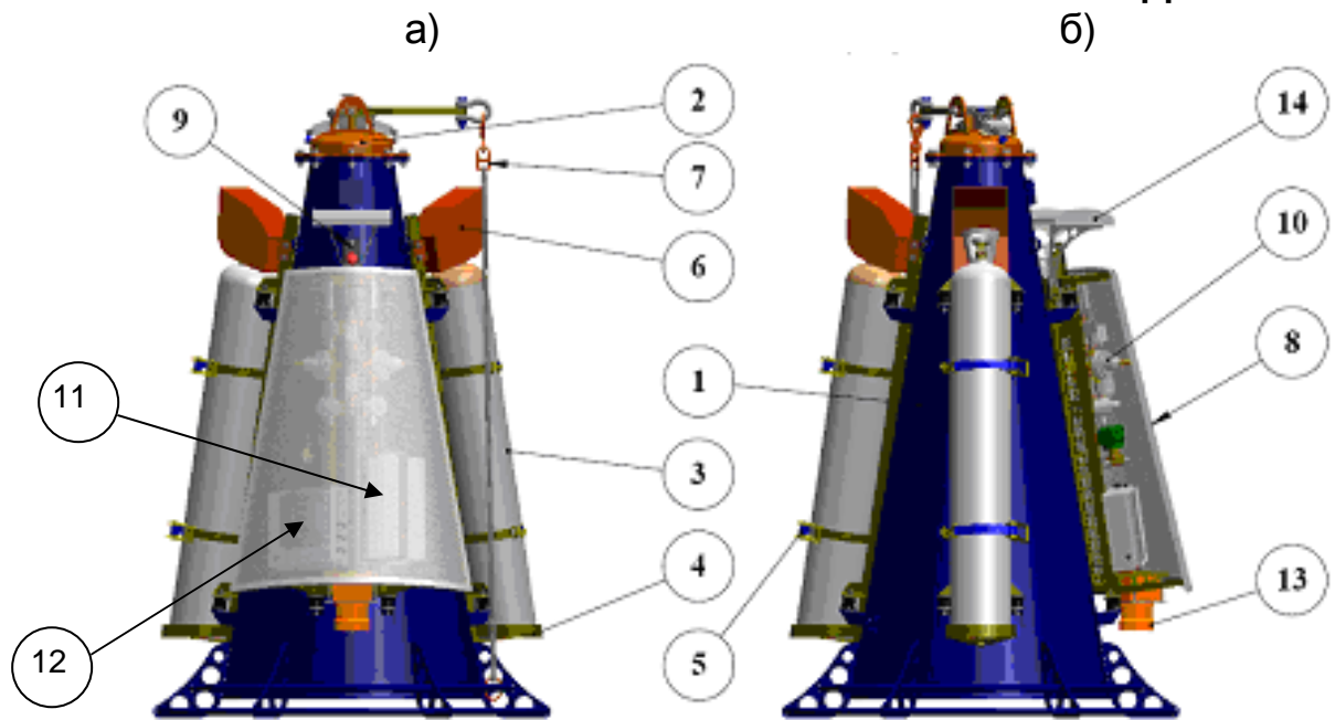
Рисунок 5.3 – Металлический конус (колокол) системы «DAISY BELL» а) – общий вид; б) – вид сбоку
