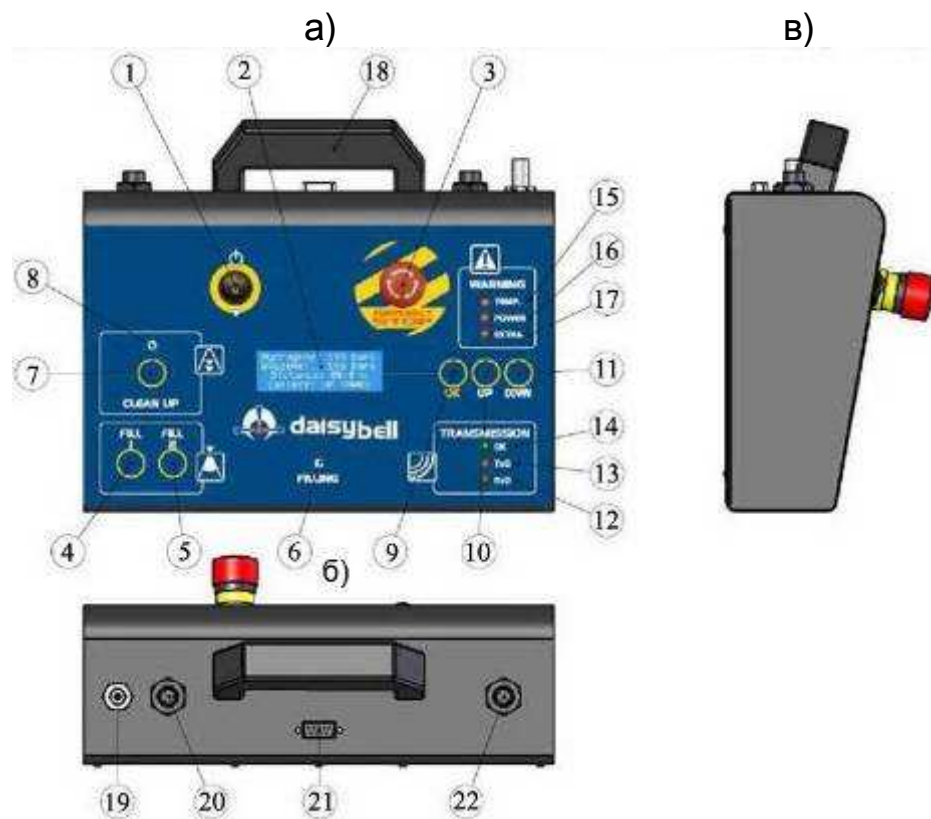
Рисунок 5.4 – Пульт управления системы «DAISY BELL» а) – общий вид; б) – вид сверху; в) – вид сбоку
